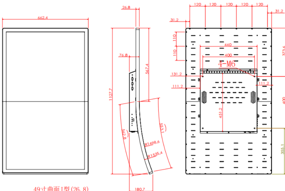
49寸曲面J型(26.8)
